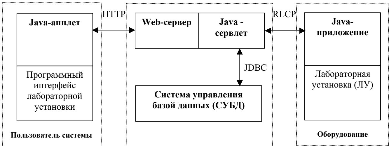
Рис.9.1. Организация доступа к удаленной лабораторной установке
